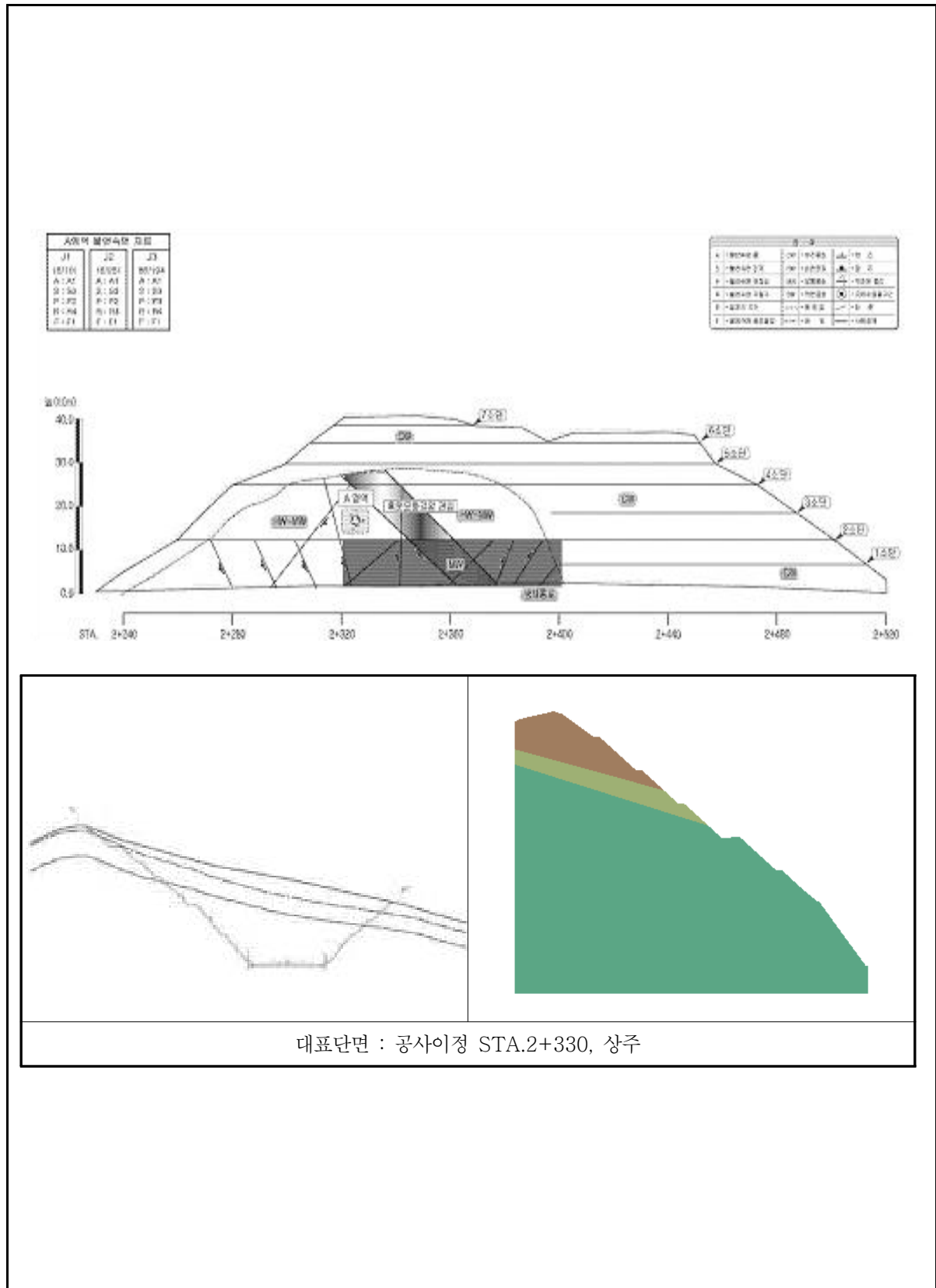
【그림 2.1.5】 표준횡단면도
